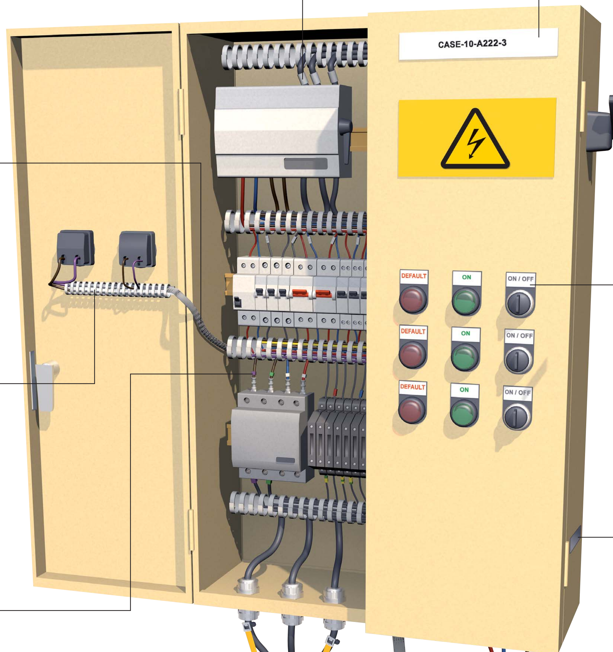
Bagues repères et plaquettes d'identification Bagues OVALGRIP et plaquettes AT
