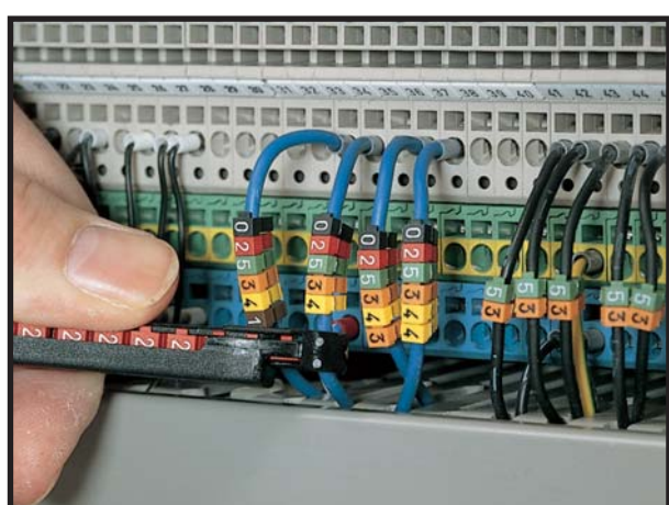
Bagues repères pré-imprimées WIC bagues ouvertes
