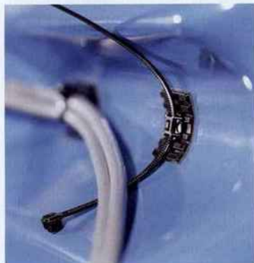
FlexTack. L'embase adhésive flexible adaptée aux surfaces concaves, convexes et angulaires.
