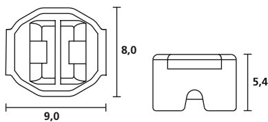
Tête de fermeture Toutes les dimensions en mm
