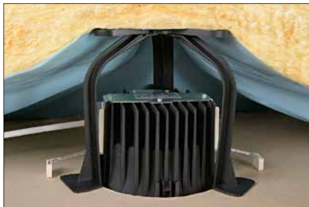
SpotClip-Kit 150 utilisé en faux plafond suspendu.
