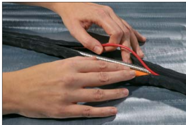
Accédez à tout moment, de manière aisée et simple aux fils et câbles pour des actions d'inspection, de maintenance et d'assemblage.
