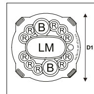
FST 13 Port Base Configuration
