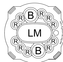
FST 13 Port Base Configuration
