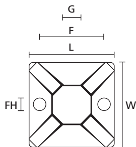
MB3-MB5 (Vue du dessus)
